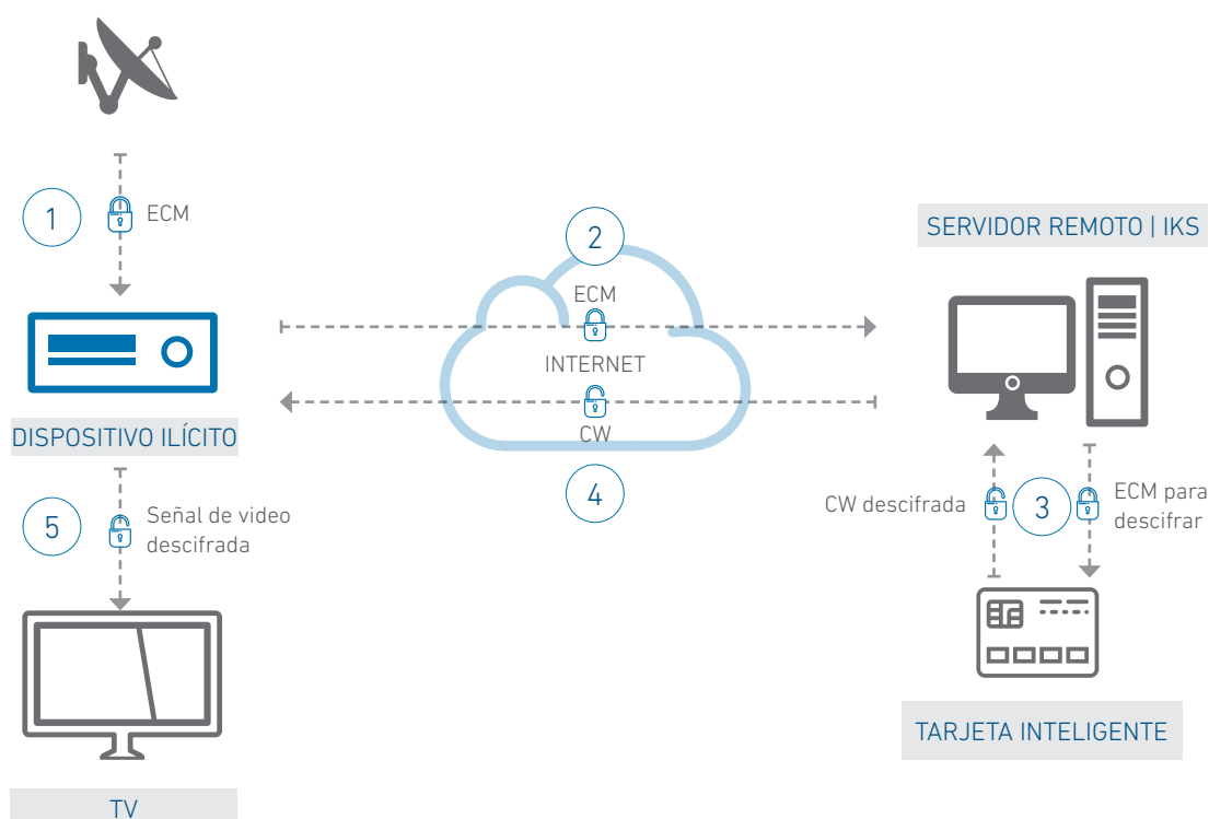
Figura 3: Arquitectura de un sistema IKS para cometer fraude
