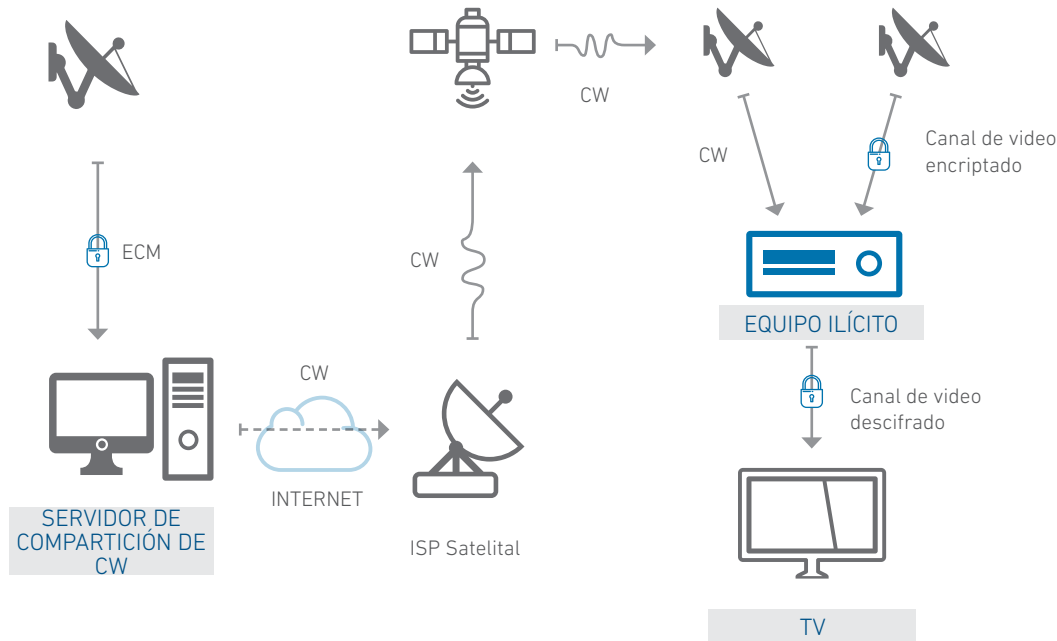
Figura 4: Arquitectura de un sistema SKS para cometer fraude
